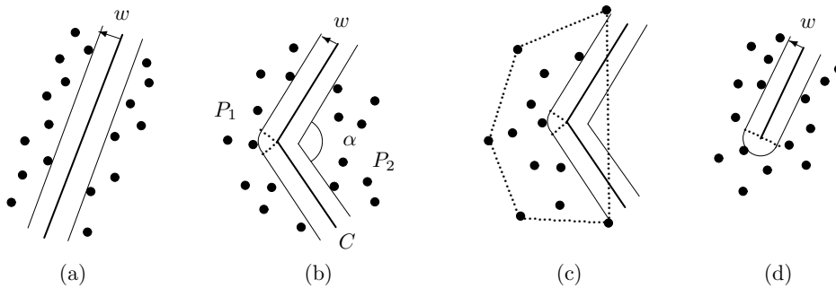
Figure 1: (a) Corridor, (b) \alpha -siphon, (c) unbounded width siphon, (d) silo
